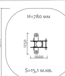
04049 Качалка на пружине "Самолет"
