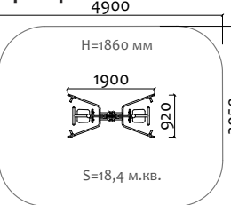
ФТ-012 Двойной тренажер для тренировки грудных мышц
