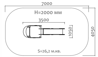
08305 Горка "Аленький цветочек"
