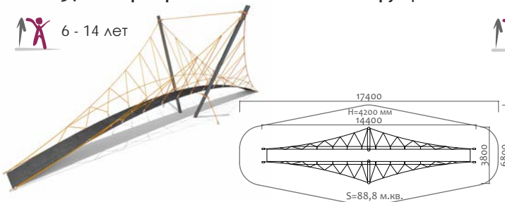
34011.21 Пространственная канатная конструкция
