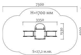
08018 Горка двойная "Морская звезда"
