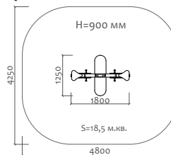
04506 Качели-балансир на пружине "Кораблик"
