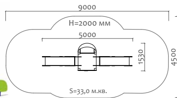
08020 Горка двойная "Морская звезда"
