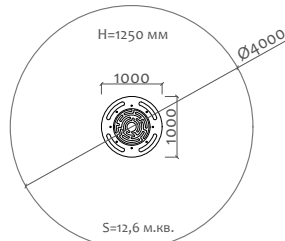
28014 Развивающий элемент "Лабиринт"
