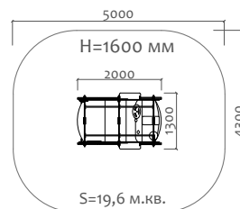
38103 Игровой элемент на пружинах "Скорая помощь"
