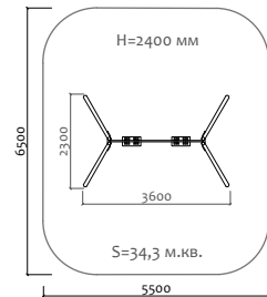
04058 Качели металлические комбинированные с подвесами
