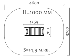
07086 Игровой элемент "Чудо-дерево"
