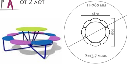
02021 Стол детский
