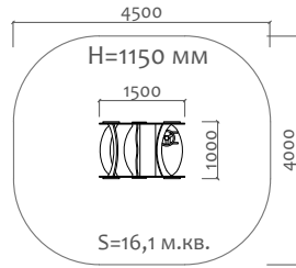
07083 Игровой элемент "Автомобиль"
