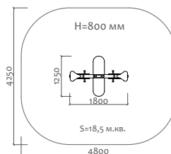
04507 Качели-балансир на пружине "Звездочка"
