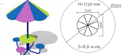
02020 Стол детский "Дубок"
