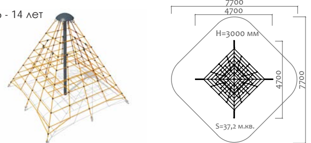
34004.21 Пространственная канатная конструкция
