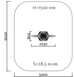
040311 Качели металлические с подвесом "Гнездо"
