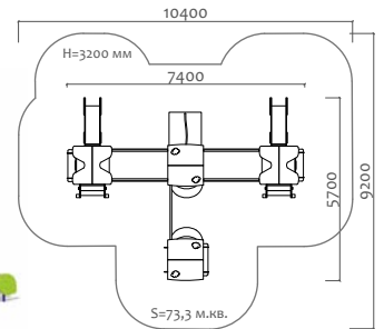
070278.21 Игровой комплекс
