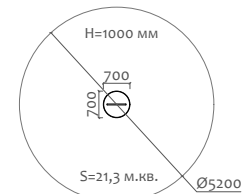
04410 Карусель с полом из резиновой крошки
