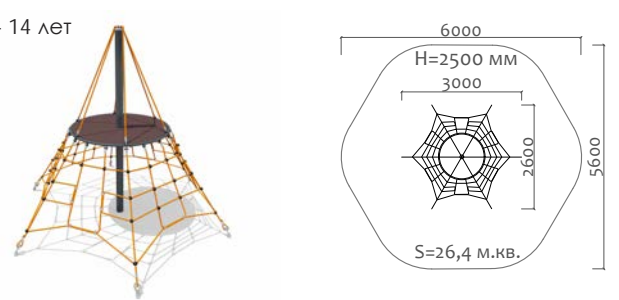
34006.21 Пространственная канатная конструкция
