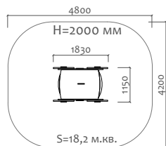
38104 Игровой элемент на пружинах "Карета"
