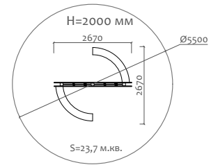
07011.21 Игровой элемент "Автобус"
