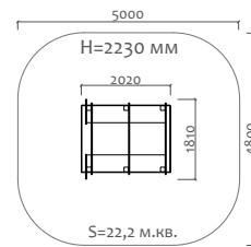
06023 Игровой элемент на пружинах "Телега"
