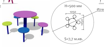
02005.21 Стол детский
