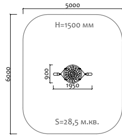
04030 Качели металлические с подвесом "Гнездо"
