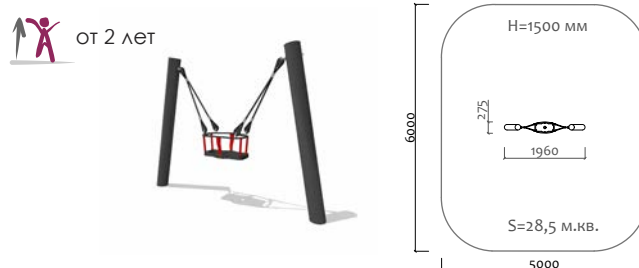
040321 Качели металлические с подвесом
