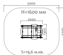
38101 Игровой элемент на пружинах "Пожарная машина"
