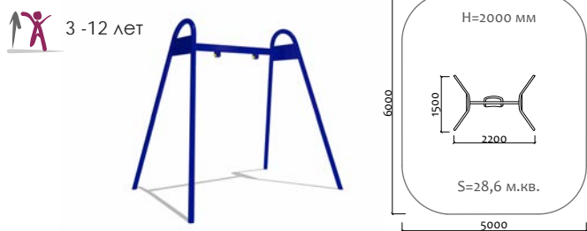
04032 Качели металлические с подвесом
