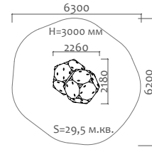
35004 Пространственная конструкция
