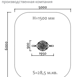
040331 Качели металлические с подвесом "Гнездо"
