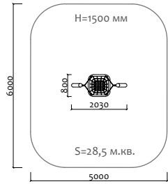
04031 Качели металлические с подвесом "Гнездо"
