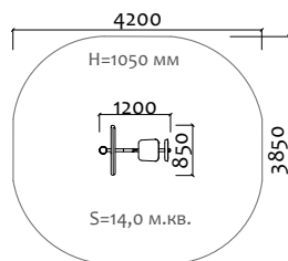
ФТ-002 Тренажер для мышц брюшного пресса
