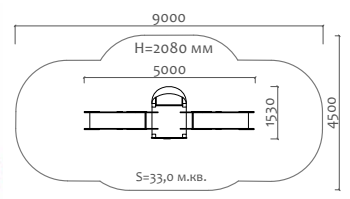
08405 Горка двойная "Аленький цветочек"
