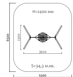
04057 Качели металлические с подвесом "Гнездо"
