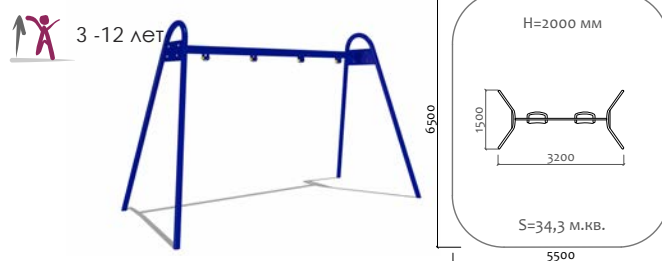
040321 Качели металлические с подвесом
