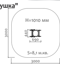
04046 Качалка на пружине "Избушка"
