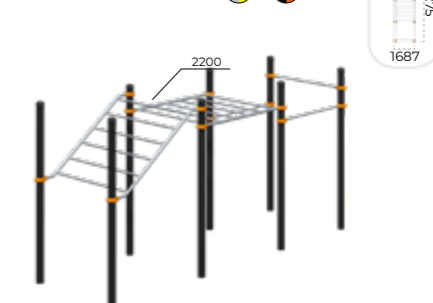
Комплекс с рукоходом Romana 501.27.01
