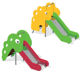
«Червяк», «Дракоша» Артикул: ИСУ-06.18.01 Артикул: ИСУ-06.19.01 Размеры ДхШхВ: 2,3x0,95x1,45 высота ската 0,8м
