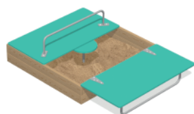
«Концепт 3» Артикул: ИСУ-05.40.02 Размеры ДхШхВ: 1,5x1,5x0,5
