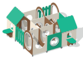
Игровой лабиринт 9 секций Артикул: ИСУ-02.24.02 Размеры ДхШхВ: 3,06x3,06x1
