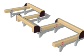
Бум-дорожка на брус Артикул: СОУ-01.46 Размеры ДхШхВ: 2,8x1x0,35
