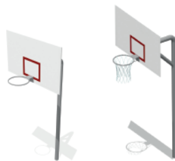
«Щит баскетбольный» детский, взрослый Артикул: СОУ-01.1 Артикул: СОУ-01.20 Размеры ДхШхВ: 1,2x0,8x1,8 Размеры ДхШхВ: 1,8x1,8x3,95
