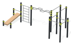
«Воркаут 6» Артикул: СОУ-02.20 Размеры ДxШxВ: 5,7x2,9x2,6
