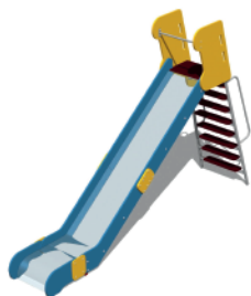
«Компакт 2» Артикул: ИСУ-06.21.01 Размеры ДхШхВ: 4x0,7x2,6 высота ската 2м
