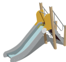
«Симпл 2» Артикул: ИСУ-06.32.01 Размеры ДхШхВ: 3,25x0,85x2,2 высота ската 1,2м
