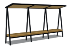
«Модульный» теневой навес 3 секции Артикул: МАФ-Н-02.02 Размеры ДхШхВ: 6,2x1,5x2,35
