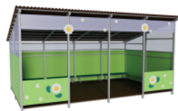
«Ромашка» металл Артикул: МАФ-02.01.22.01 Размеры ДхШхВ: 6х4,2х3,2 Полезная площадь: 21 м 2
