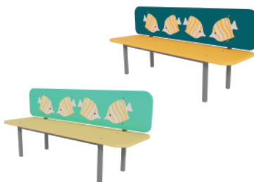
«Рыбки» Артикул: МАФ-СД-05.00 Размеры ДхШхВ: 1,2х0,37х0,7
