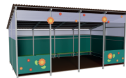
«Гербера» металл Артикул: МАФ-02.01.22.02 Размеры ДхШхВ: 6х4,2х3,2 Полезная площадь: 21 м 2
