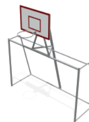
Ворота с баскетбольным щитом (с сеткой) Артикул: СОУ-01.37 Размеры ДхШхВ: 3,2x1,85x3,3
